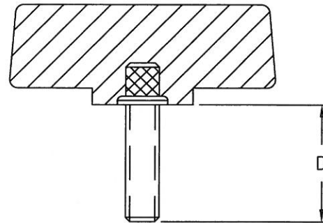
THREADED STUD
