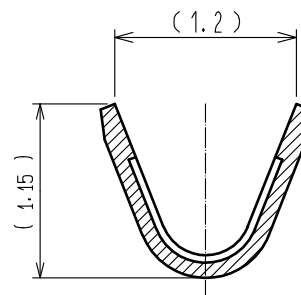
A-A(20:1)
