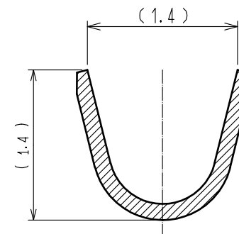
B-B(20:1)
