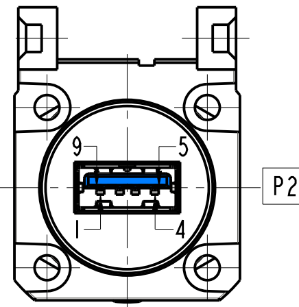
USB3.0-A Vue B avant sans bouchon Front view B without cap Affectation des broches / Pin assignments
