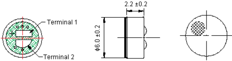
Dimensions : Millimetres
