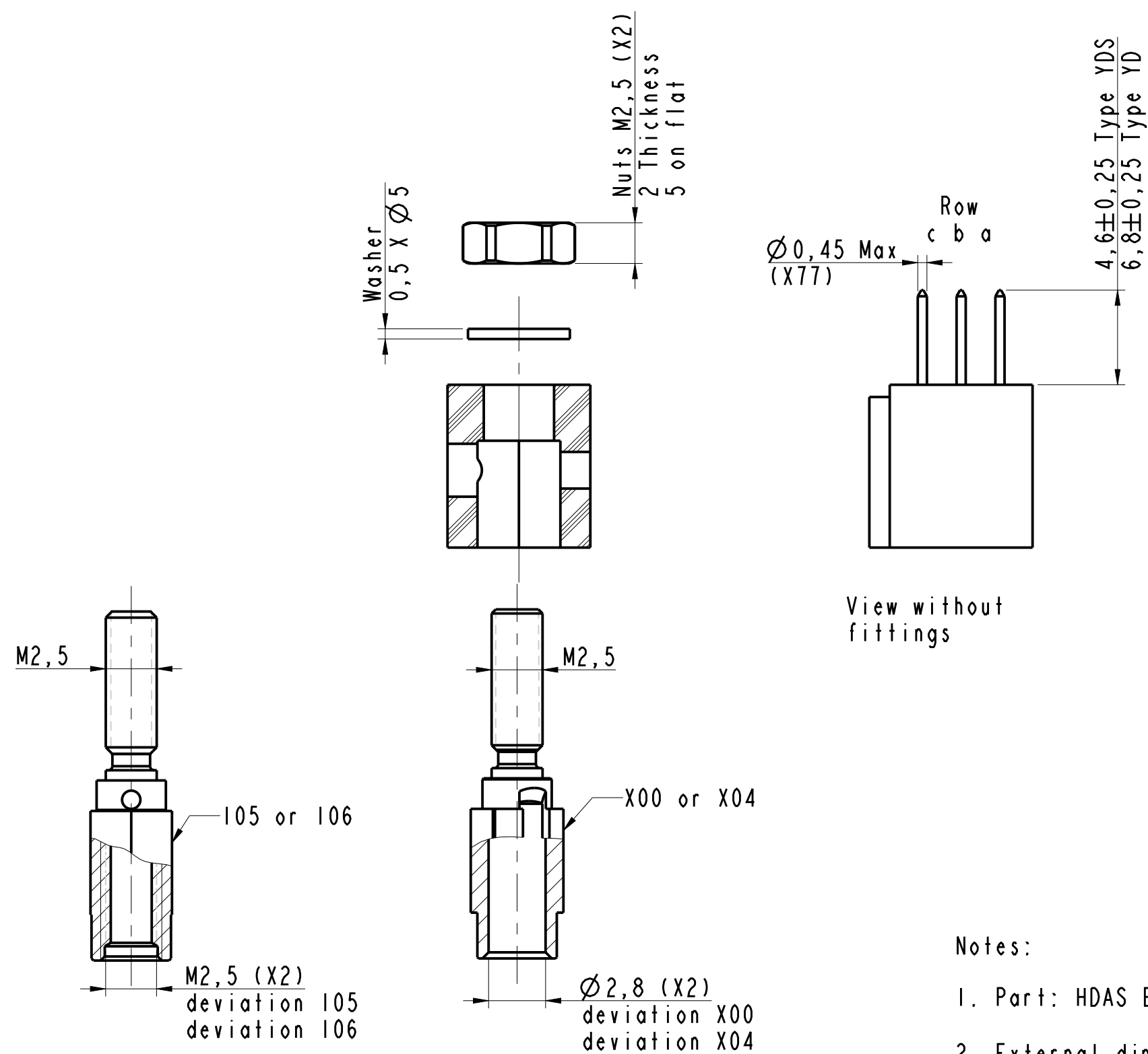
Section A-A
