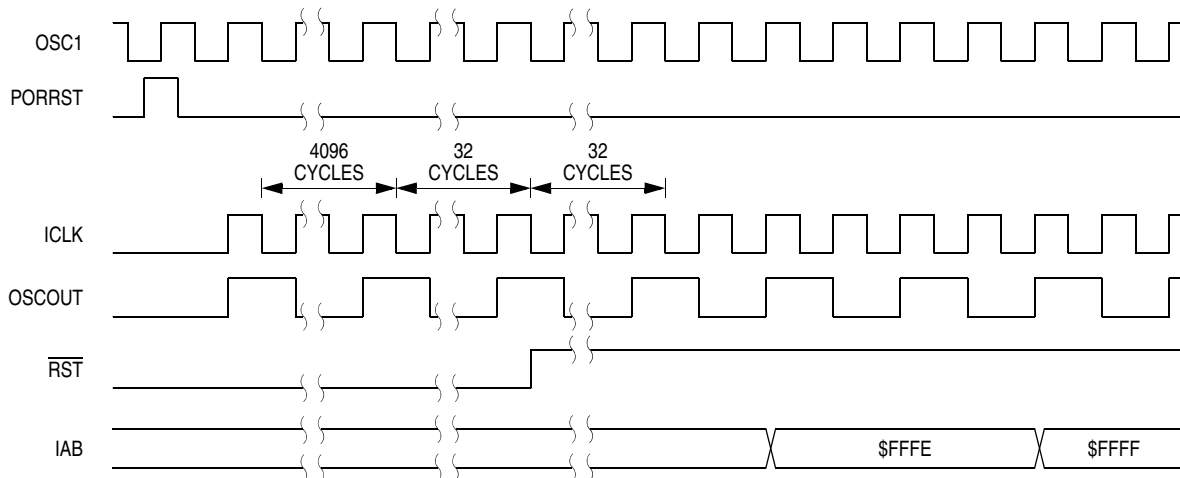
Figure 5-7. POR Recovery
