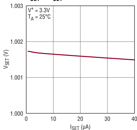
V_{\text{SET}} vs I_{\text{SET}}
