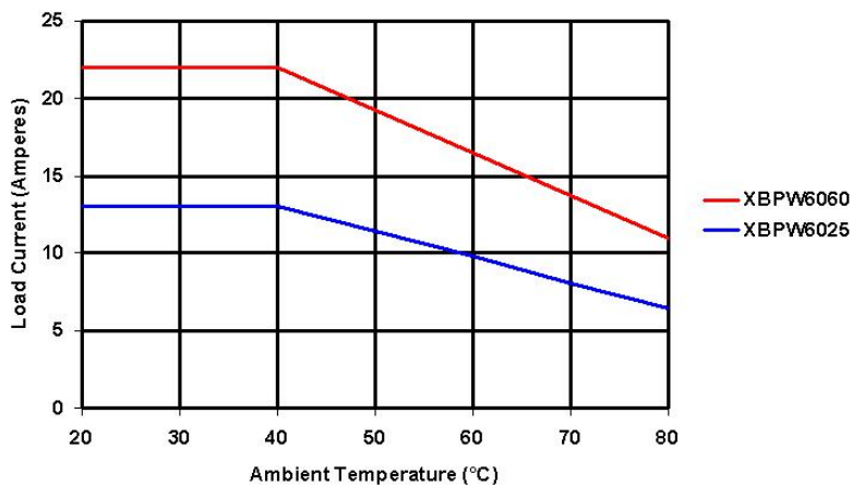
HS271DR w/25A or 60A SSR
