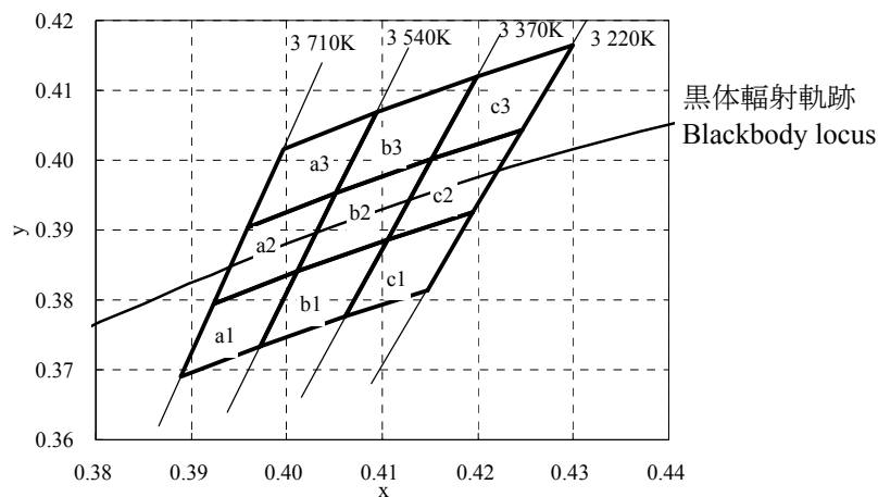
色度図 Chromaticity diagram
