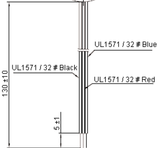
Dimensions : Millimetres
