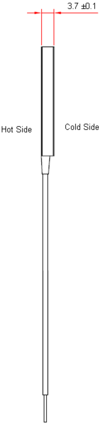
Dimensions : Millimetres
