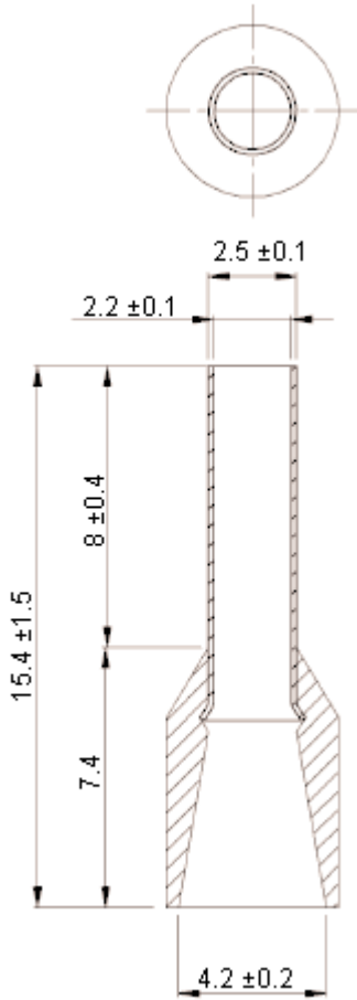
Dimensions : Millimetres
