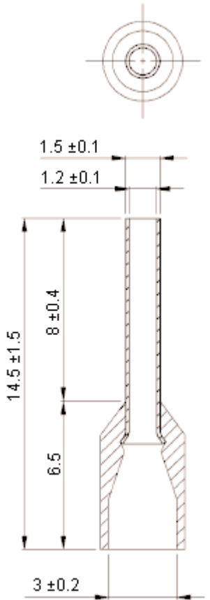
Dimensions : Millimetres
