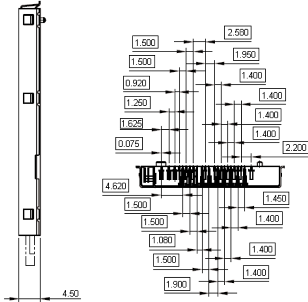
Dimensions : Millimetres
