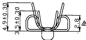
Dimensions : Millimetres
