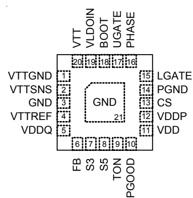
WQFN-20L 3x3
