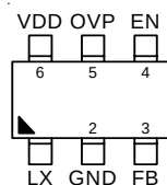
TSOT-23-6
