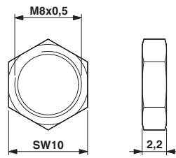
Flat nut M8
