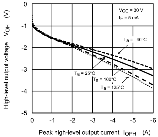
Fig. 12.2.10 V_{OH} - I_{OPH}
