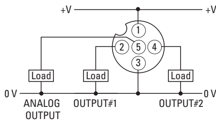
Circuit diagrams E76-CLR...
