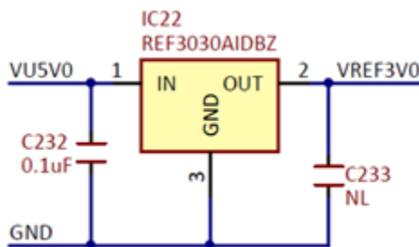
Figure 17. VREF3V0 .
