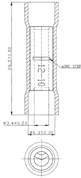
Dimensions : Millimetres
