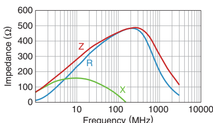
MMZ1608R150A
