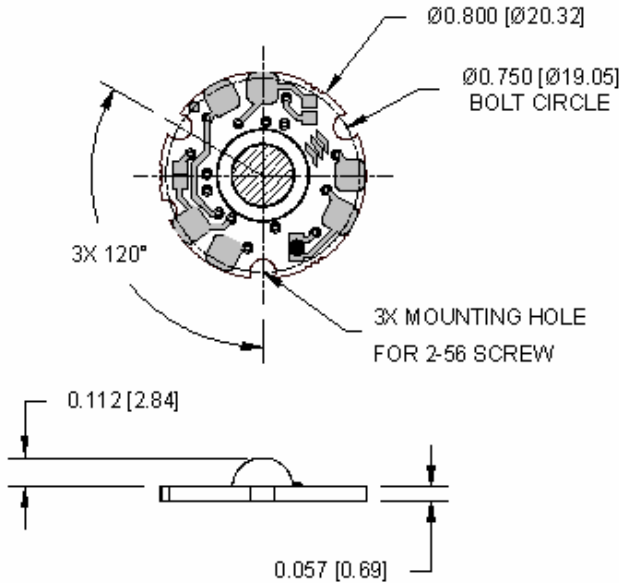
ATLAS RGB, P/N NT-43F0-0424
