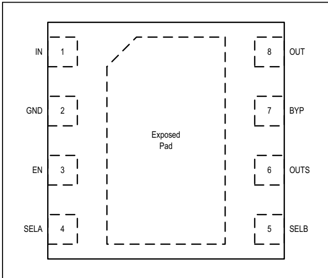
MAX38902A
