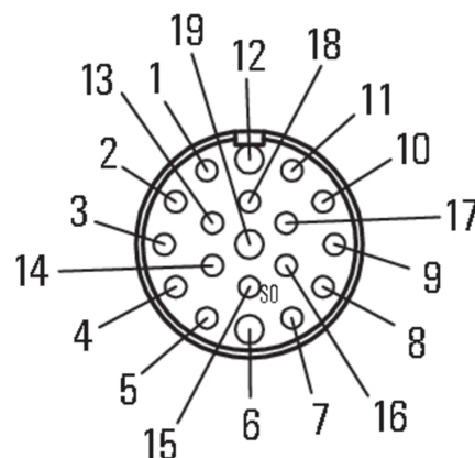
Connecteur femelle
