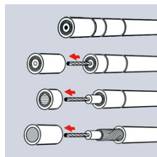
Pelado de cables coaxiales en 3 pasos
