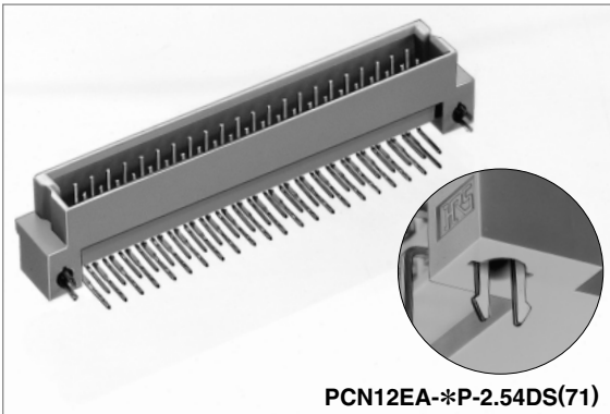
PCN12EA- P -2.54DS(71)
