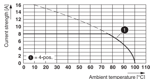
Type: MC 1,5/ 4-ST-3,81 with MCV 1,5/ 4-ST-3,81
