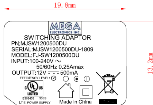
比例/Scale: 3:1
