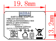
比例/Scale: 1:1
