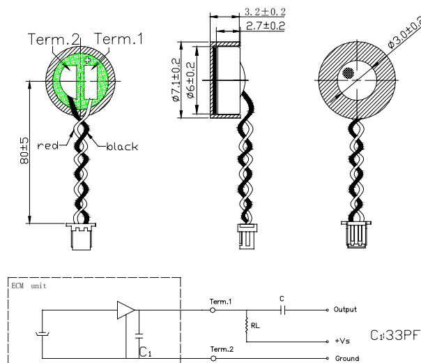
Dimensions : Millimetres
