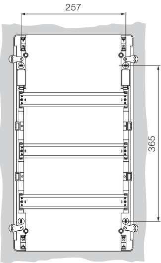
36 modules
