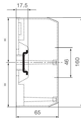
4-6 modules
