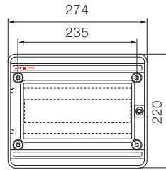
12 modules
