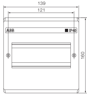
6 modules
