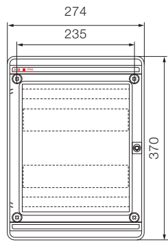
24 modules
