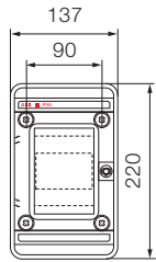
4 modules
