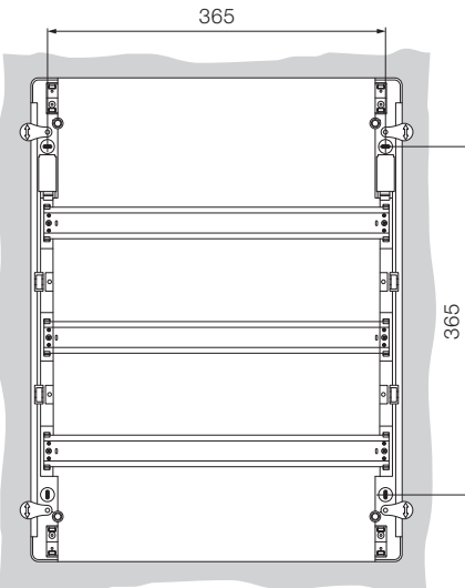
54 modules
