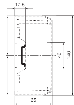
2 modules
