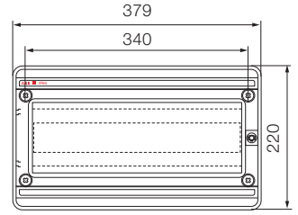
18 modules
