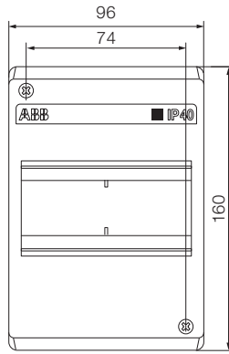
4 modules
