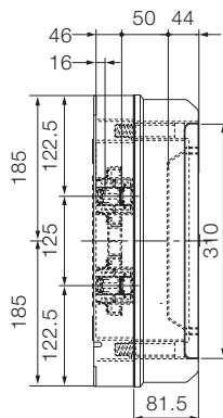
24 modules
