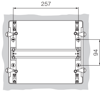
12 modules
