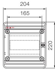
8 modules
