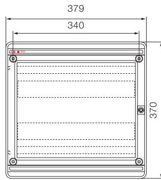
36 modules
