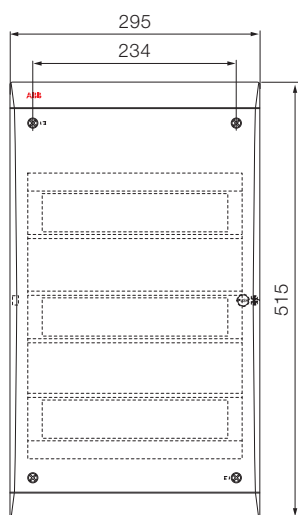
36 modules
