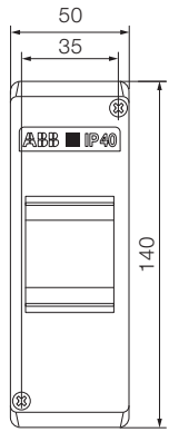
2 modules
