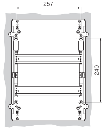
24 modules
