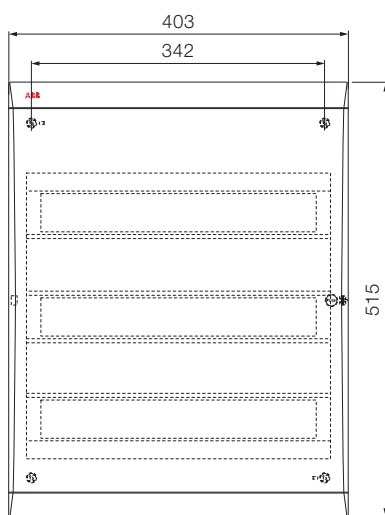
54 modules
