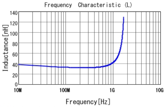
■ LQG15HS33NJ02 L
