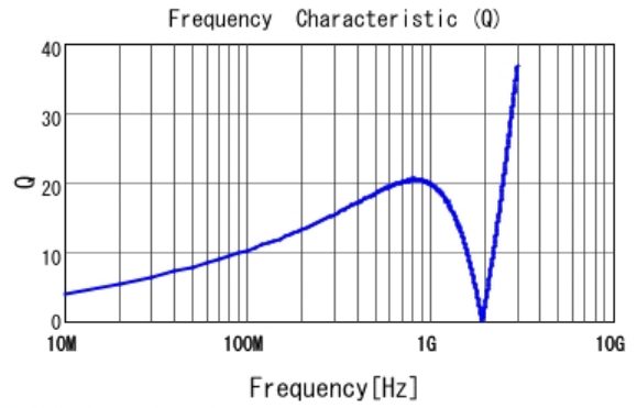
■ LQG15HS33NJ02 Q
