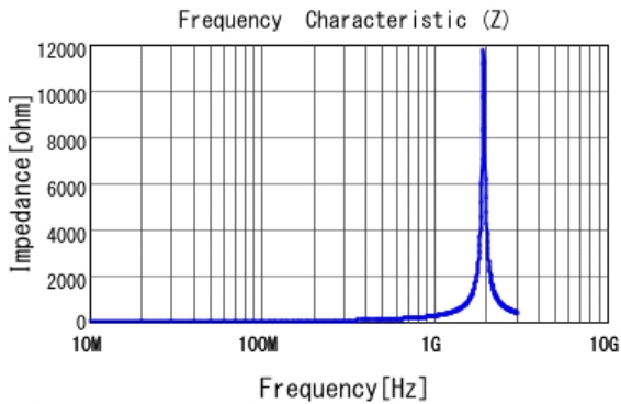
■ LQG15HS33NJ02 |Z|
