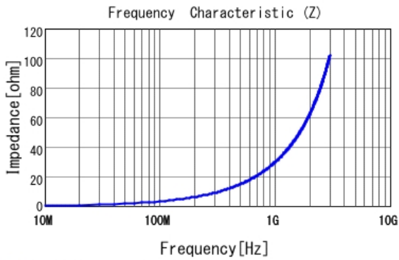
■ LQP03TN4N7H02 |Z|
