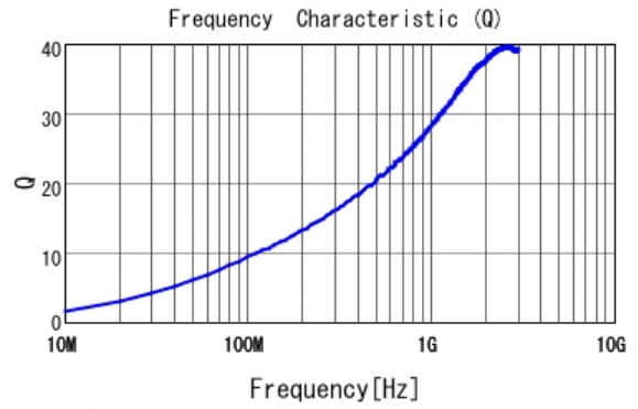
■ LQP03TN4N7H02 Q
