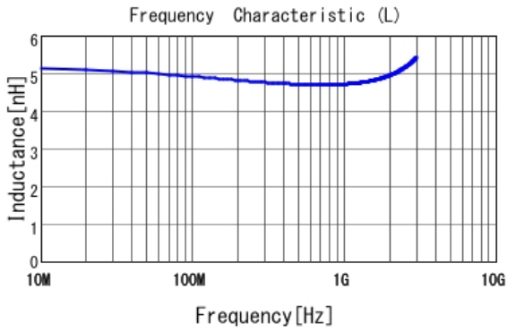
■ LQP03TN4N7H02 L
