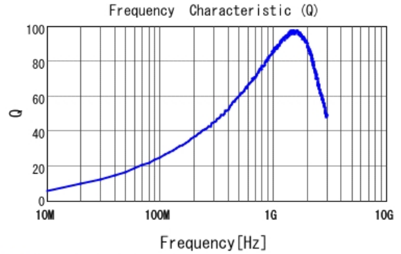
■ LQW18AN18NJ00 Q
