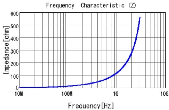
■ LQW18AN18NJ00 |Z|
