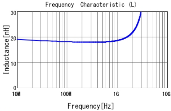
■ LQW18AN18NJ00 L
