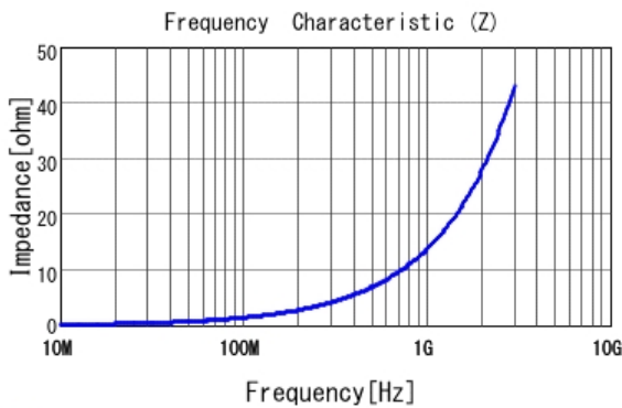
■ LQW18AN2N2C80 |Z|
