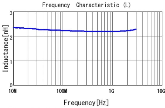
■ LQW18AN2N2C80 L
