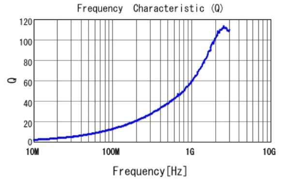
■ LQW18AN2N2C80 Q
