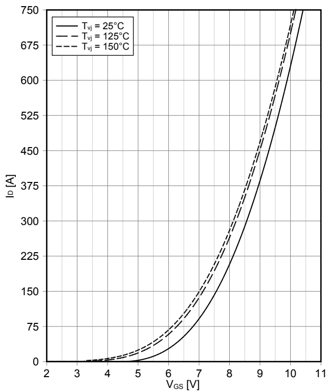
Übertragungscharakteristik MOSFET (typisch) transfer characteristic MOSFET (typical)
