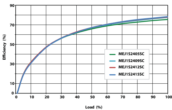
24V Input
