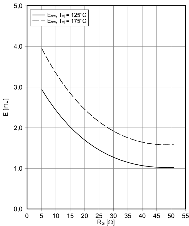
Schaltverluste Diode, Wechselrichter (typisch) switching losses Diode, Inverter (typical) E_{rec} = f(R_G) I_F = 50 \text{ A}, V_{CE} = 600 \text{ V}
