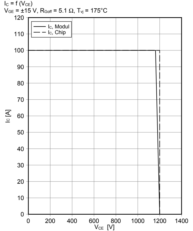
Sicherer Rückwärts-Arbeitsbereich IGBT, Wechselrichter (RBSOA) reverse bias safe operating area IGBT, Inverter (RBSOA) I_C = f(V_{CE}) V_{GE} = \pm 15 \text{ V} , R_{Goff} = 5.1 \Omega , T_{vj} = 175^\circ\text{C}
