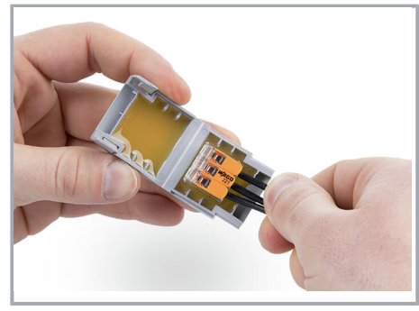
Verdrahtete Klemme in die Gelbox einlegen.
