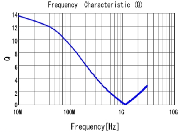
■ LQW18CAR27J00 Q
