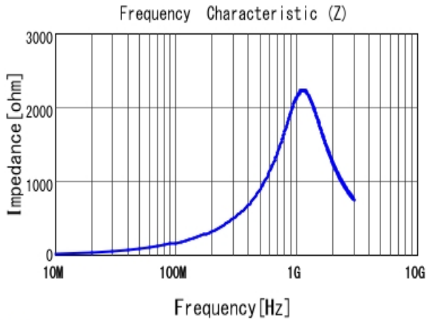
■ LQW18CAR27J00 |Z|
