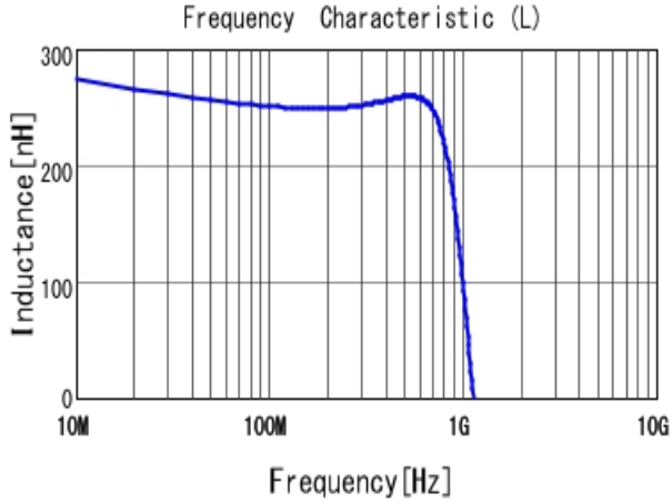
■ LQW18CAR27J00 L
