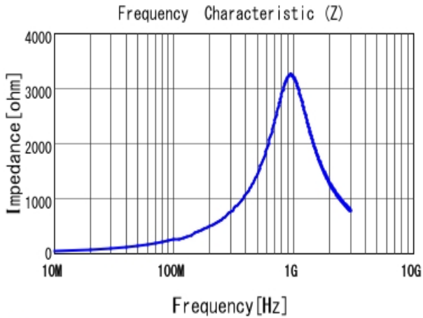
■ LQW18CAR40J00 |Z|
