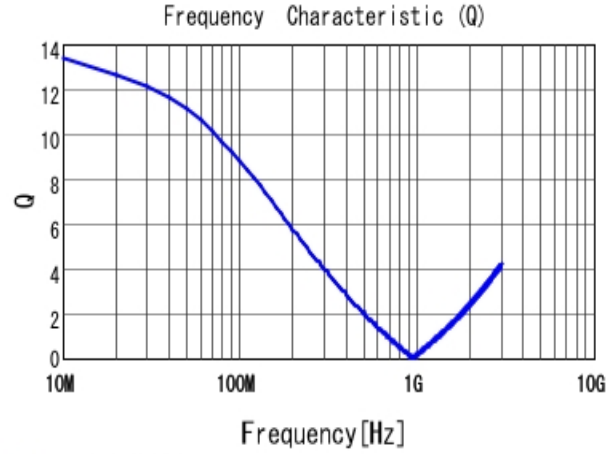
■ LQW18CAR40J00 Q
