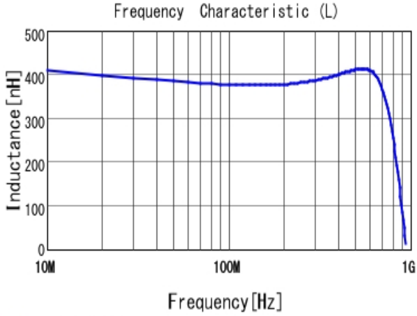
■ LQW18CAR40J00 L
