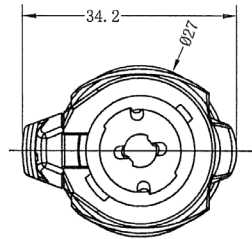
Dimensions : Millimetres
