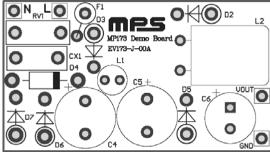
Top layer
