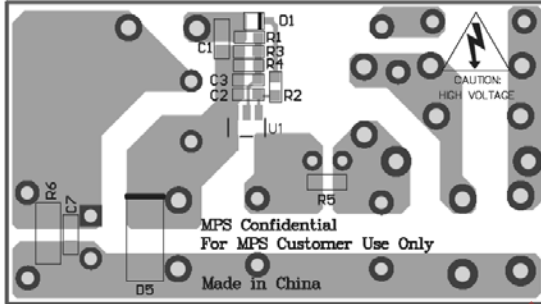
Bottom layer
