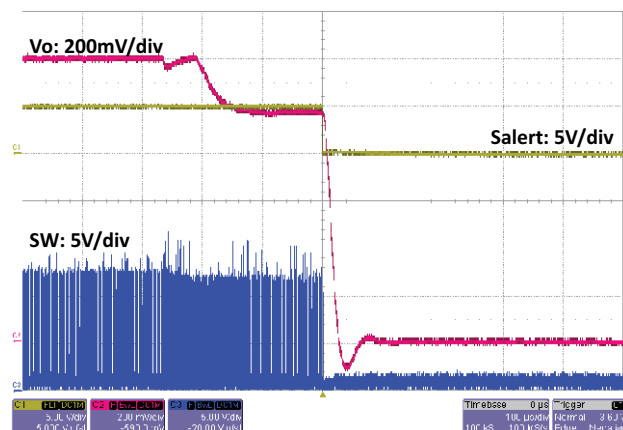
Fig. 34 - SiC451 UVP
