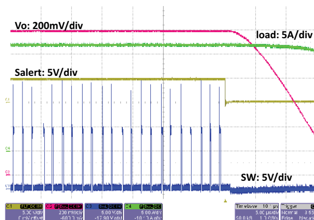
Fig. 15 - SiC453 OCP
