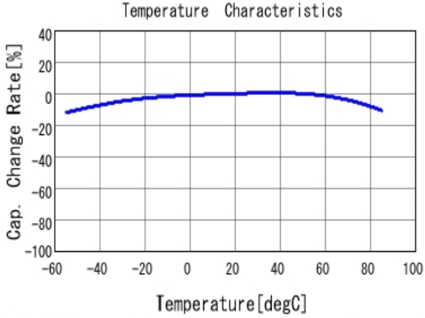
■ GRM188R60J226MEA0 C-Temp. capchange, DCO. 0V, ACO. 1Vrm
