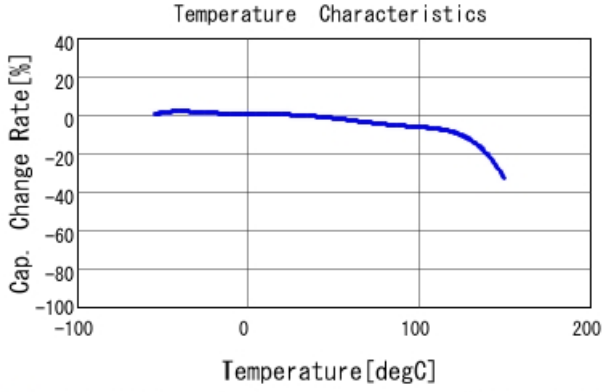
■ GCJ188L8EL104KA07 C-Temp. capchange, DCO. 0V, AC1. 0Vrm
