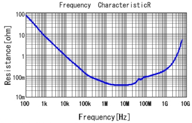
■ GCJ188L8EL104KA07 R DCOV, 25degC
