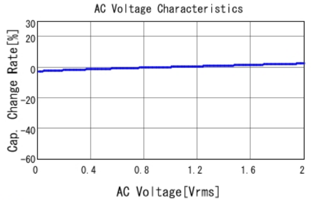
■ GCJ188L8EL104KA07 C-AC Voltage capchange, DCOV, 25.0d
