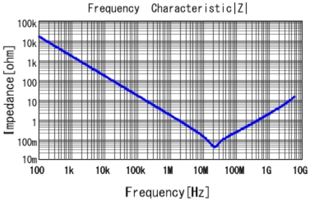
■ GCJ188L8EL104KA07 |Z| DCOV, 25degC
