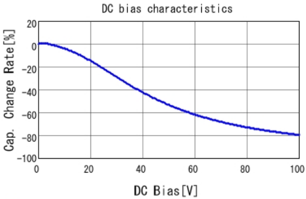
■ GCJ188L8EL104KA07 C-DC bias capchange, 25.0degC, AC1.
