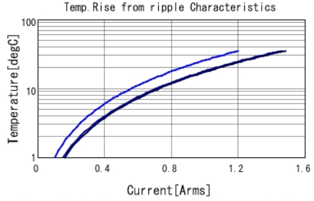
■ GCJ188L8EL104KA07 Temp. rise ■ 400kHz ■ 800kHz ■ 1MHz
