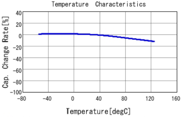
■ KCM55WR71E476MH01 C-Temp. capchange, DCOV, ACO. 5Vrms
