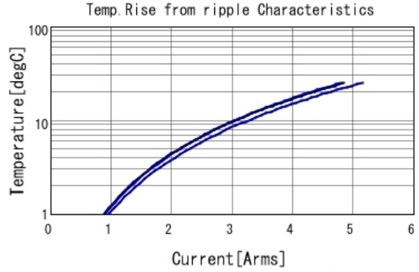
KCM55WR71E476MH01 Temp. rise ■ 50kHz ■ 100kHz ■ 300kHz
