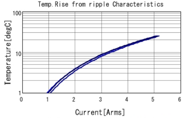
KCM55WR7YA336MH01 Temp. rise ■ 50kHz ■ 100kHz ■ 300kHz
