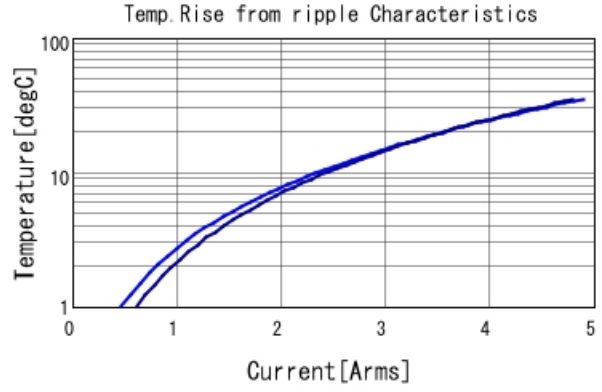
GRM188R61E106KA73 Temp. rise ■ 400kHz ■ 800kHz
