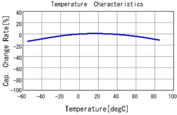
■ GRM188R61E106KA73 C-Temp. capchange, DCO. 0V, ACO. 2Vrm
